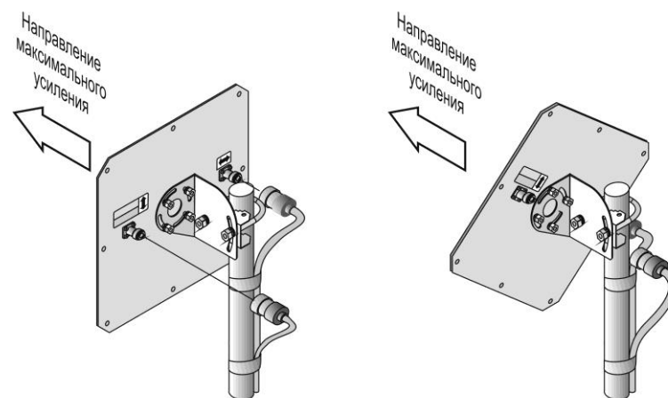
Рисунок 2. Сборка антенны
