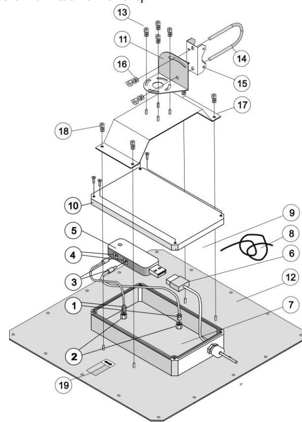
Рисунок 3. Сборка антенны
