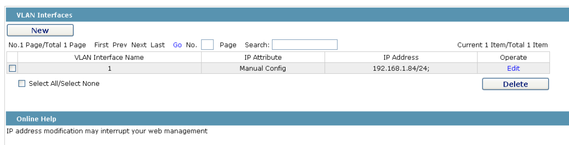
Рисунок 2: Настройка интерфейса VLAN
